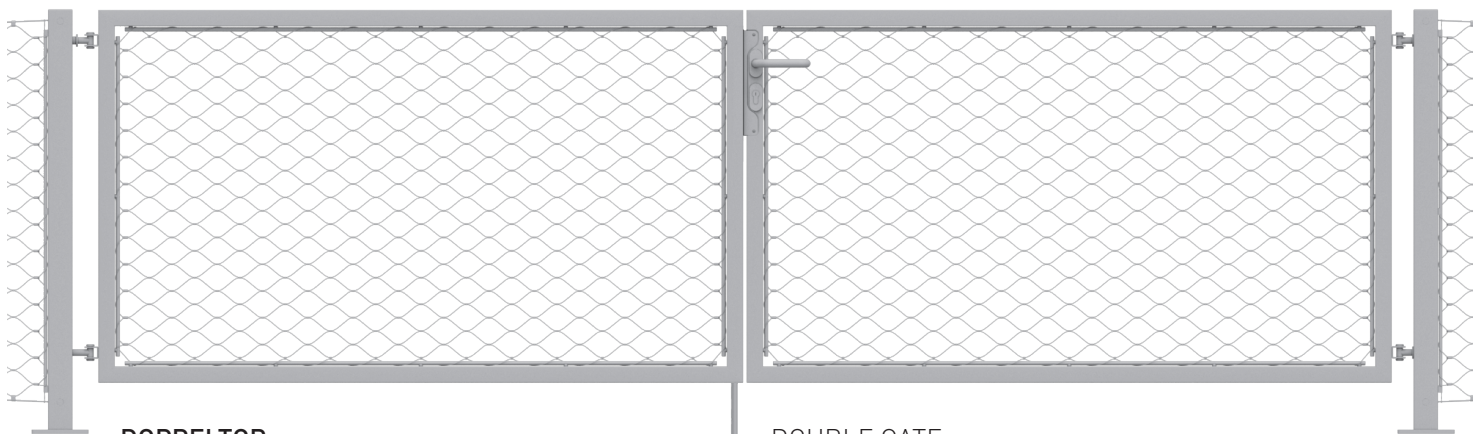
DOPPELTOR mit Öffnung nach innen. Durchgang 3200 mm
