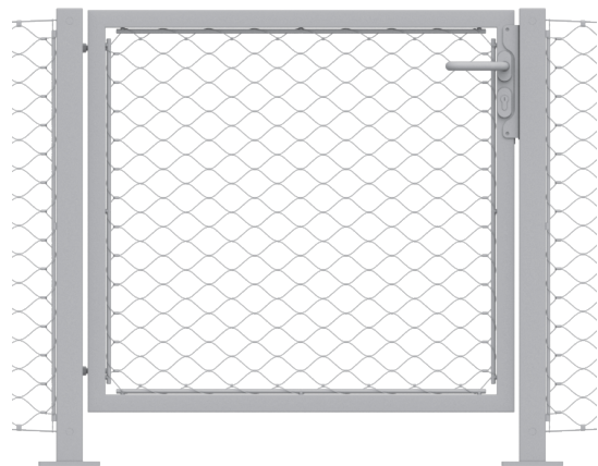
EINZELTOR mit Anschlag links oder rechts und Öffnung nach innen. Durchgang 1000 mm
